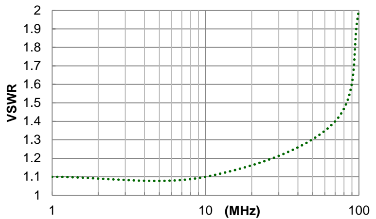
Output VSWR
