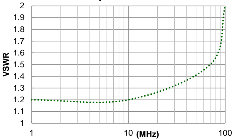
Input VSWR
